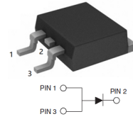
TO-263AB
