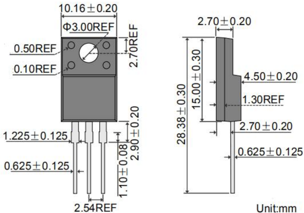
ITO-220AB
